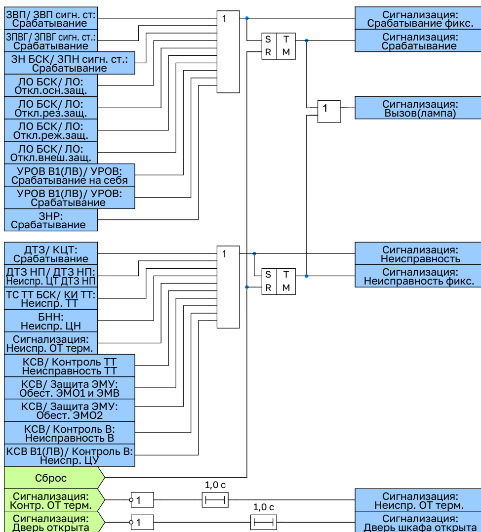
Рисунок 2.33 – Функциональная схема логики блока сигнализации
