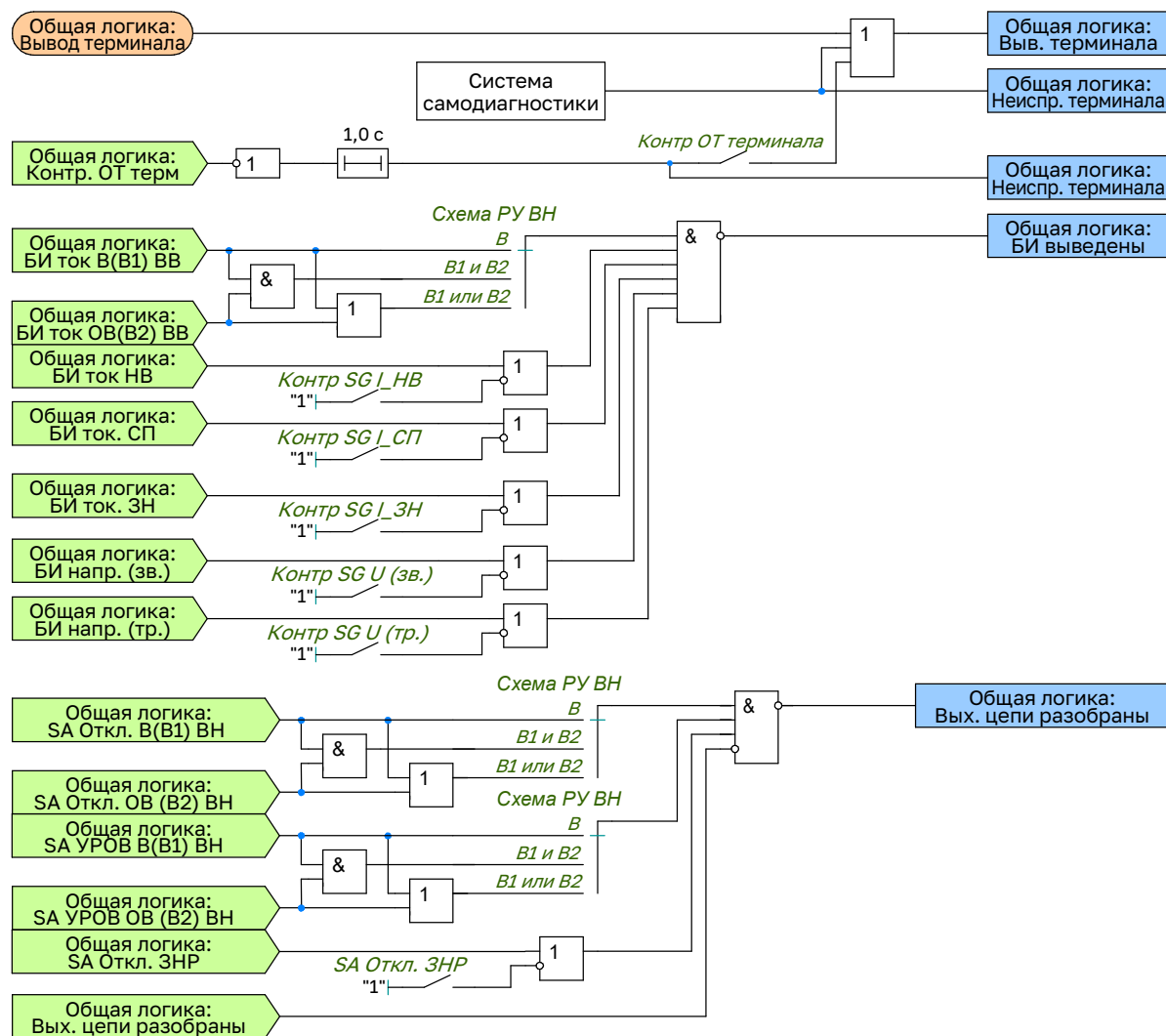
Рисунок 2.34 – Функциональная схема общей логики
